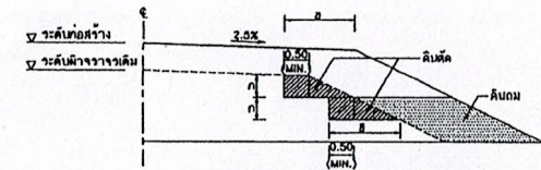
รูปตัดการก่อสร้างลาดคันค้ำทางบนถนนเดิม
